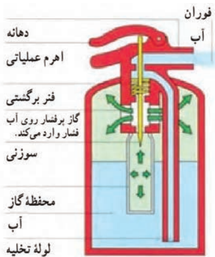
شکل ۳-۵ خاموش‌کننده دستی حاوی آب
