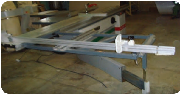
شکل ۵-۴۹- میله‌کشویی جلوی میز متحرک برای برش صفحات بزرگ
