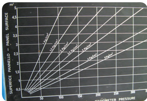
شکل ۵-۸۱- دیگرام یا منحنی رابطه بین سطح و فشار در یک پرس روغنی
