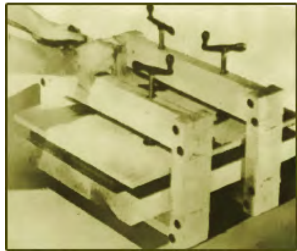
شکل ۱-۶- پرس دستی اولیه، که صفحات کمکی، به وسیله‌ی کلاف‌های کمک، پیچ و مهره و دسته‌ی همدلی عمل پرس‌کاری را انجام می‌داد.
