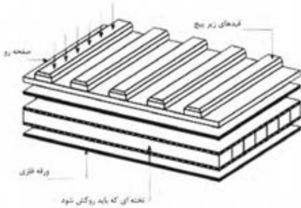
شکل ۳-۶- با قرار دادن صفحات کمکی کمک بر رو و زیر صفحه‌ی مورد نظر، عمل پرس‌کاری انجام می‌شود.
