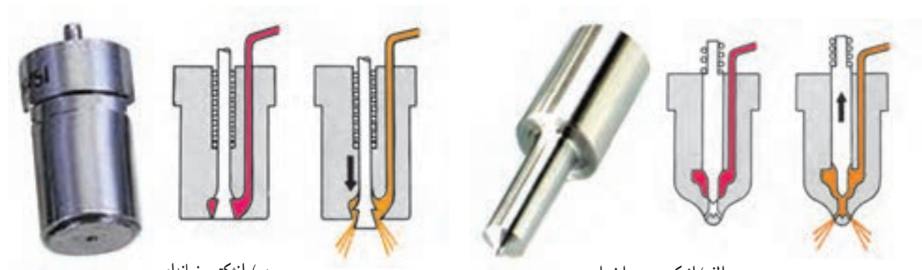
شکل ۱۷-۴- انواع انژکتور
