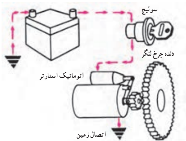
شکل ۶-۴۵- ورود جریان به اتوماتیک استارتر
