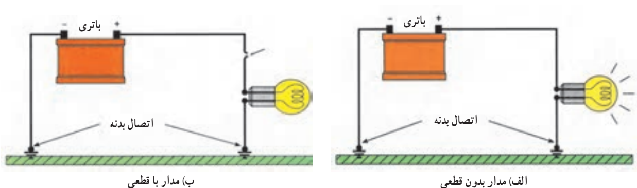
شکل ۷۱-۶ وضعیت قطعی در یک مدار ساده
