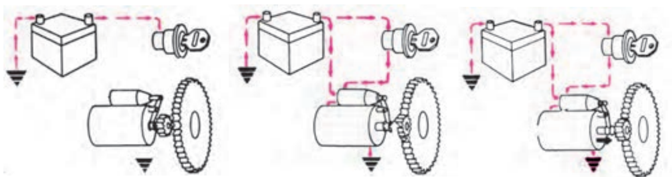
شکل ۴۸-۶- برگشت دنده استارت به عقب
