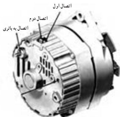
شکل ۲۶-۶- آلترناتور
