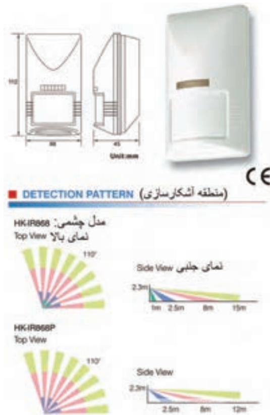
شکل ۱۲-۲ منطقه دید دو نوع چشمی با لنز استاندارد
