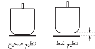
شکل ۳۷-۵- فاصله‌ی بین نوار و شکاف هد
