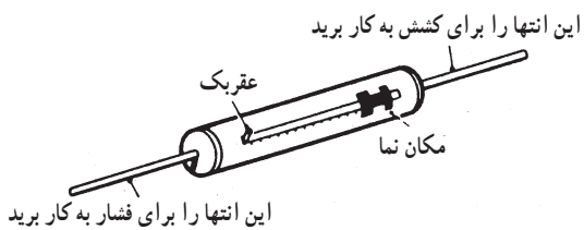
شکل ۴۶-۵- ترازوی فنری
