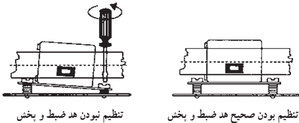
شکل ۵-۳۳ پیچ تنظیم زاویه ی جانی هد
