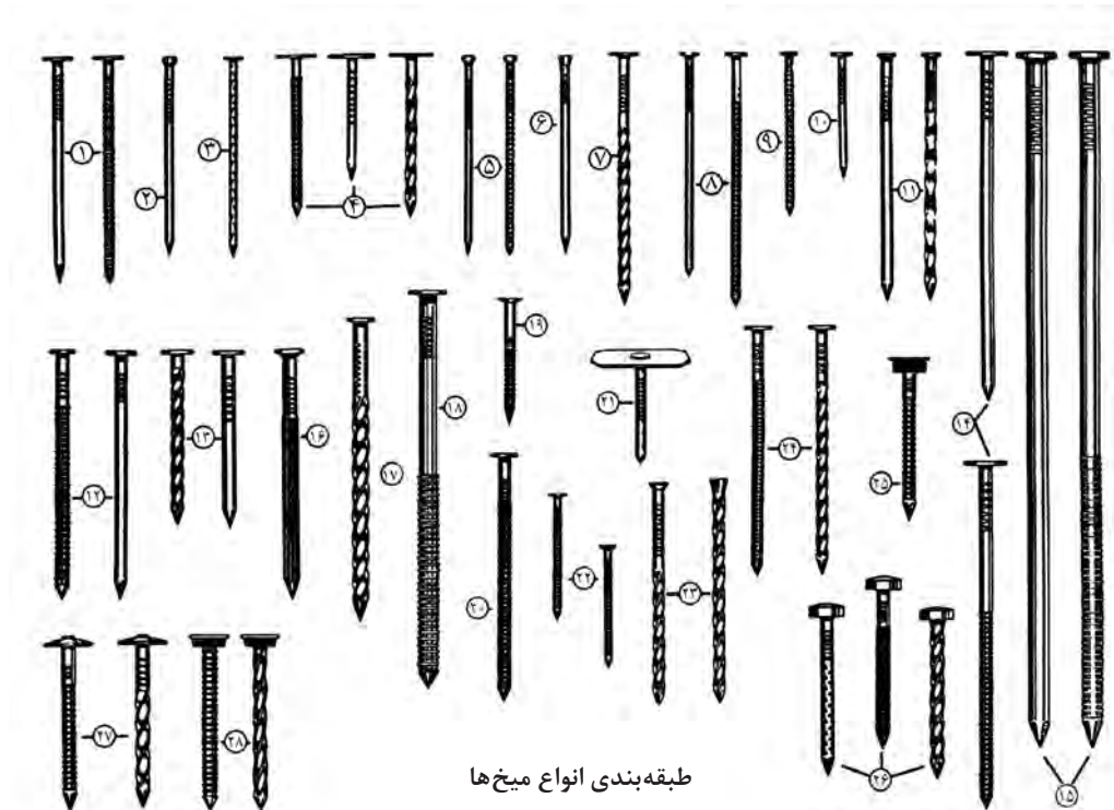
شکل ۵- طبقه‌بندی انواع میخ‌های رزوه دار که باعث افزایش مقاومت برشی میخ در چوب می‌شود.
