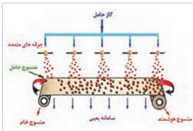
شکل ۱۳- دو سامانه نانومقیاس تولید و تکمیل افشانه‌ای نانوذرات بر روی پارچه
