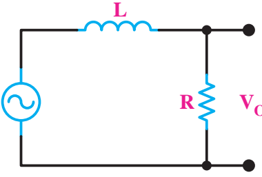
فیلتر پایین گذر RL
