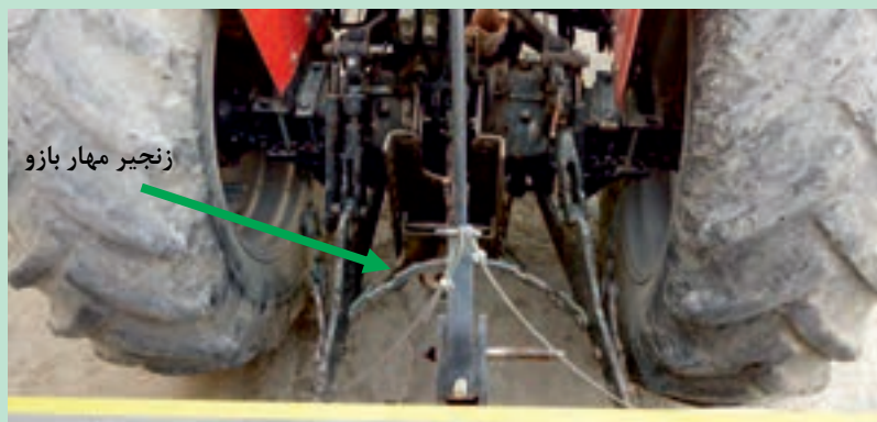
شکل ۱۴ - زنجیر مهار بازوی تراکتور
