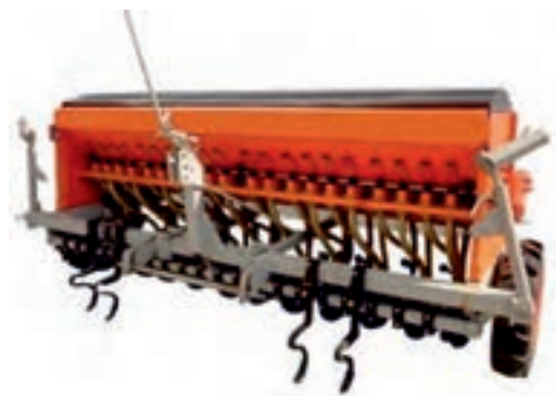
شکل ۴- خطی کار جهت کاشت غلات با قابلیت تنظیم جهت کاشت ریز دانه
