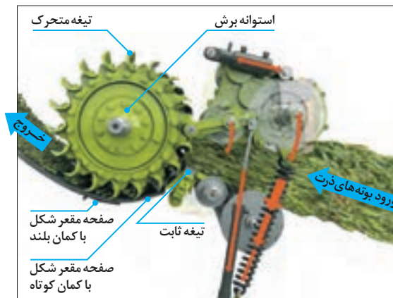
شکل ۱۹- واحد برش
