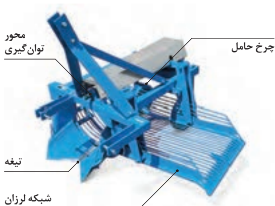
شکل ۱۰- سیب زمینی کن لرزان
