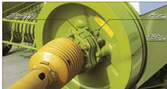
شکل ۸۰- چرخ لنگر و کلاچ ایمنی
