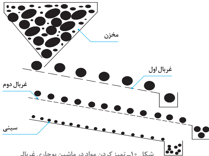
شکل ۱۰- تمیز کردن مواد در ماشین بوجاری غربالی
