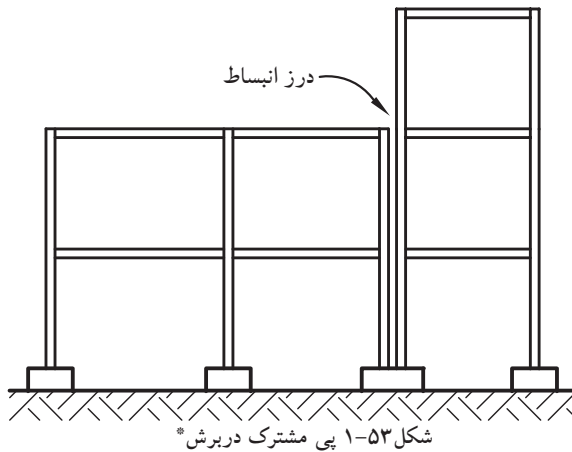
* در این برش، پناهی بار وارده‌ی متغیر، نیاز به پی باسکولی ۱ است تا پی مورد نظر تعادل و ایستایی خود را حفظ نماید.
