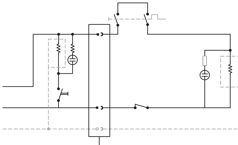
شکل ۲۴-۱ مدار الکتریکی چای ساز معمولی
