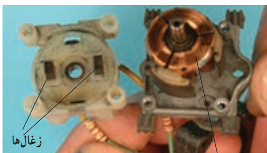
تیغه‌ی کلکتور
