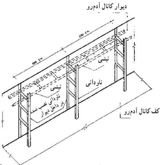
الف - جزئیات تیپ اسکله بندی نصب کابل در داخل کانال‌های آدمرو دیوار کانال آدمرو
