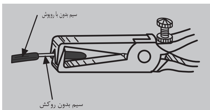
شکل (۱-۲۸) سیم لخت کن ساده
