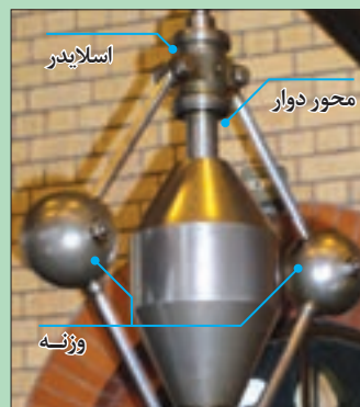
شکل ۱۴- گاورنر
