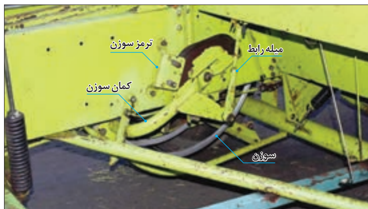
شکل ۵۴- اجزای قسمت سوزن ها
