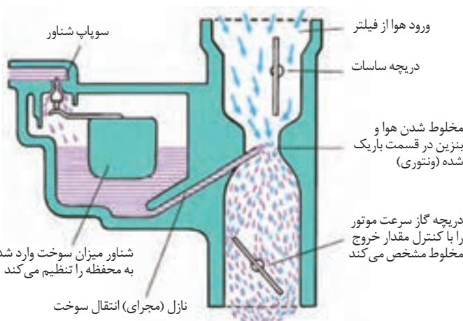
شکل ۱۰- نحوه کار کاربراتور
