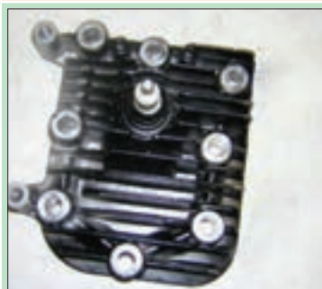
۸- سر سیلندر را پیاده کرده و پیچ‌های آن را به ترتیب در محل رسم شده روی کارت بچینید.
