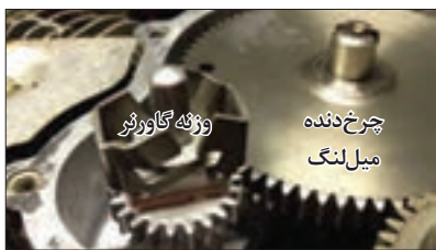
شکل ۱۳- وزنه‌های گاورنر
