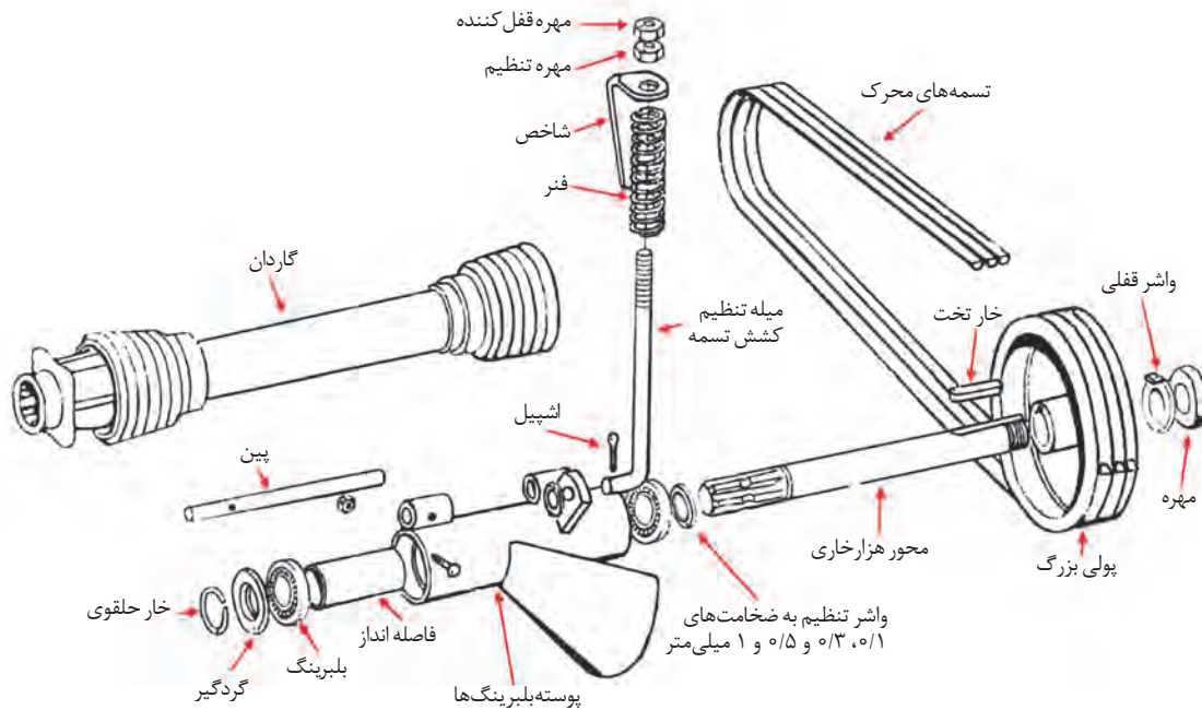
شکل ۱- اجزای انتقال قدرت به چرخ تسمه بزرگ یک نمونه دروگر استوانه‌ای ساخت ایران
