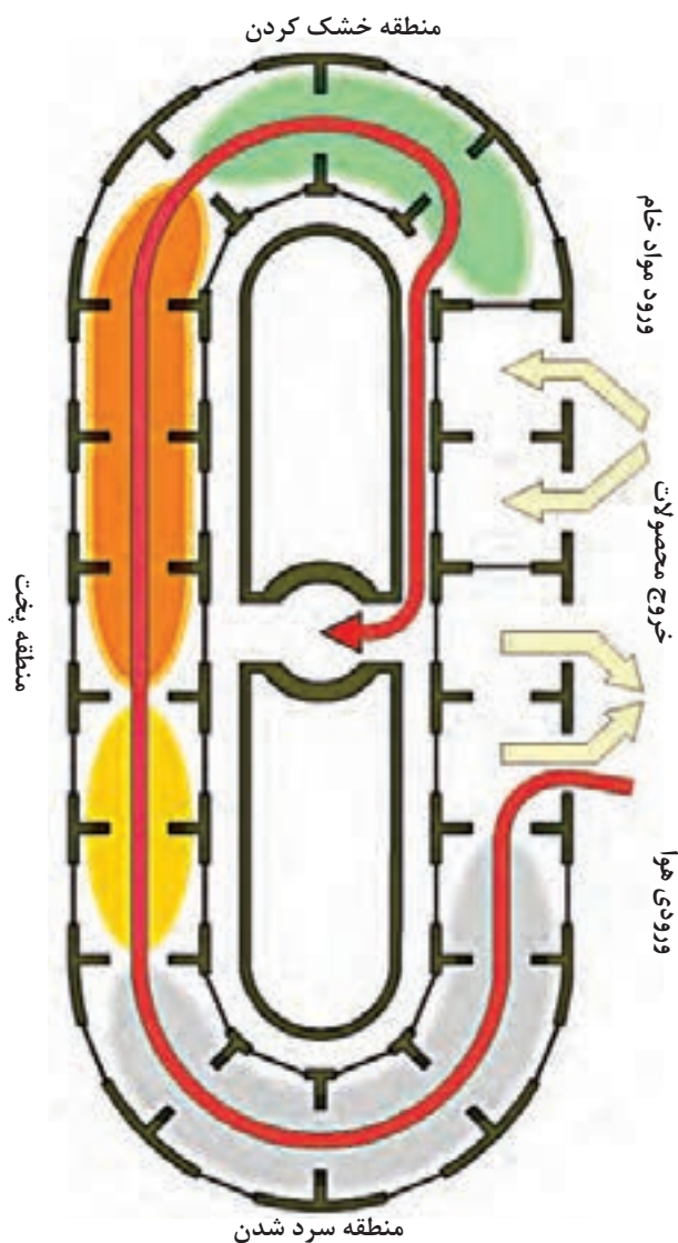
شکل ۱۳- کوره هوفمن
