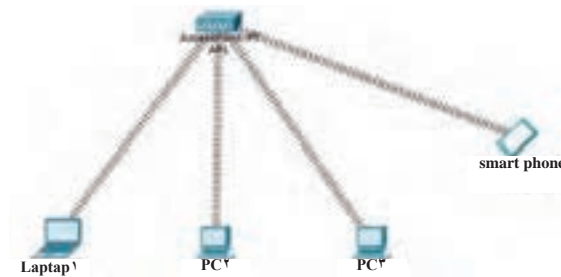
شکل ۱۷- شبکه InfraStructure
