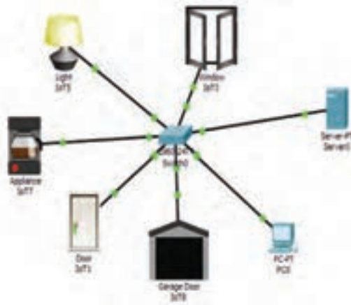
شکل ۴۳- اینترنت اشیا
