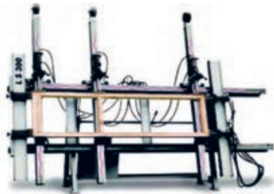
شکل ۴۳- نمونه‌ای از ماشین مونتاز کلاف
