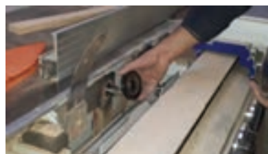
شکل ۶۲- باز کردن مهره و فلنج جلوی تیغه
