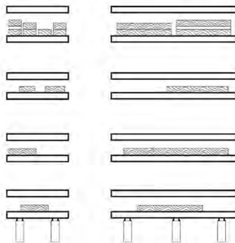
شکل ۴۰- چیدمان غلط قطعه کار زیر پرس
