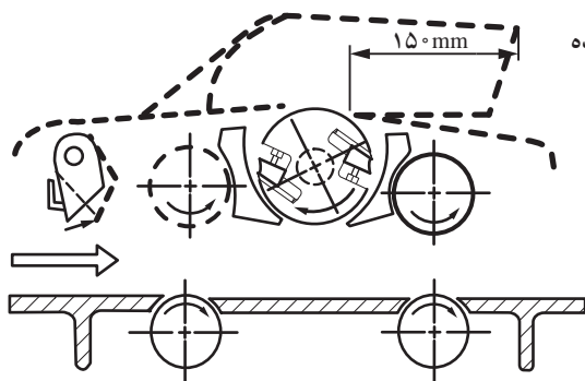
شکل ۲۸- درجه تنظیم میزان باردهی ماشین کف رند
