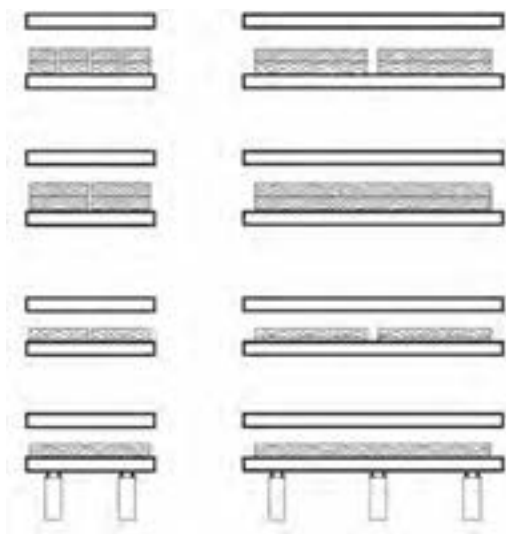
شکل ۴۱- چیدمان صحیح قطعه کار زیر پرس
