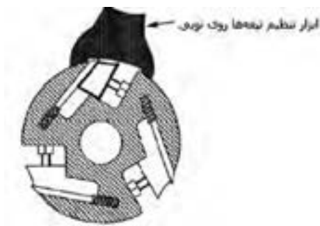
شکل ۲۷- روش تعویض تیغه رنده و نحوه قرار گرفتن تیغه و استقرار آن روی تویی
