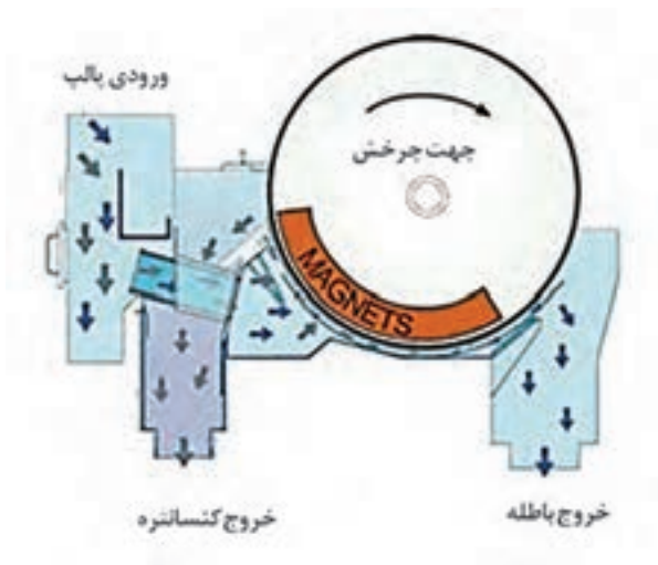
شکل ۲۹- با گردش استوانه غیر هم جهت
