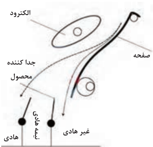
شکل ۳۸- دستگاه جدا کننده الکترواستاتیکی صفحه ای
